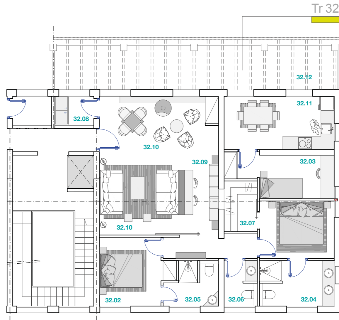
Nid 32 Escala 1:100
